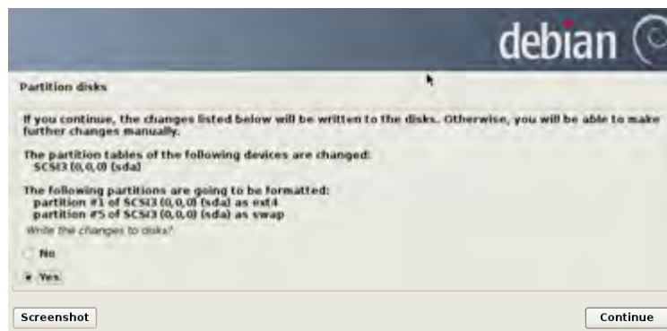
Gambar 8.20. Konfirmasi tentang partisi untuk menginstall
